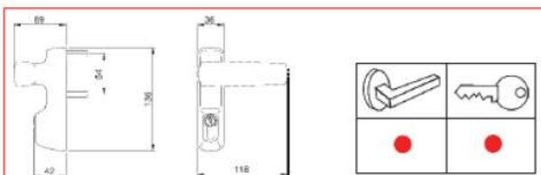
Massimo spessore della porta mm 105
