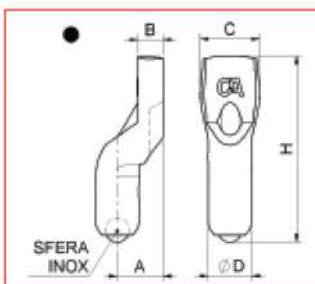
PERNO SFERICO INFERIORE CON SFERA INOX, ZINCATO
