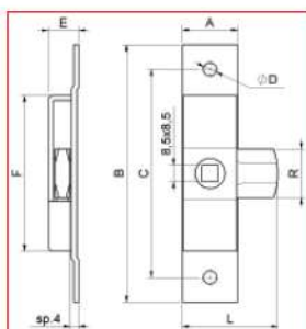
CHIAVISTELLO A SCATTO PER SPORTELLI ZINCATO
