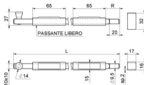
CATENACCIO VERTICALE 10x10 CON PUNTA TONDA, ZINCATO
