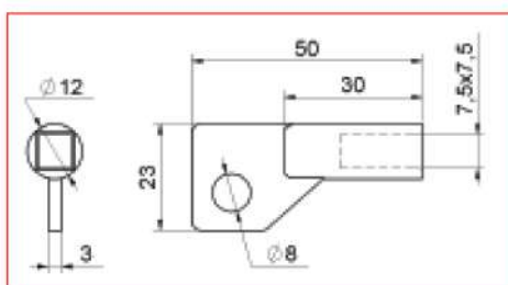
CHIAVE QUADRA PER TAVELLINO
