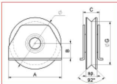
RUOTA GOLA A V A 1 CUSCINETTO, SUPPORTO LATERALE, ZINCATA
