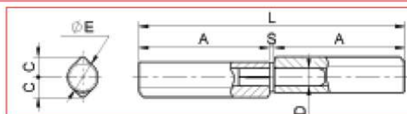
CERNIERA STAMPATA 2 ALI A COSTA, PERNO E RONDELLA FISSA IN ACCIAIO
