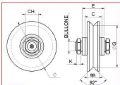
RUOTA GOLA A V A 1 CUSCINETTO, CON INGRASSATORE, ZINCATA
