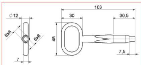
CHIAVE PER CHIAVISTELLO
