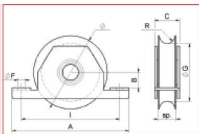
RUOTA GOLA A H A 1 CUSCINETTO, SUPPORTO INTERNO, ZINCATA
