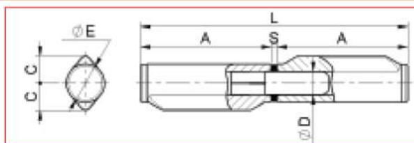
CERNIERA STAMPATA 2 ALI A COSTA, PERNO FISSO IN ACCIAIO RONDELLA SFILABILE IN OTTONE
