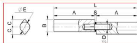
CERNIERA A GOCCIA TORNITA, PERNO OTTONE CON CUSCINETTO
