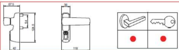
Massimo spessore della porta mm 105
