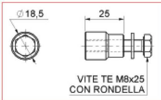
ATTACCO A SALDARE PER CREMAGLIERA RETTANGOLARE ZINCATA
