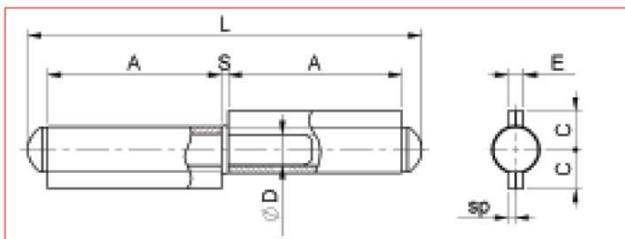
CERNIERA TRANCIATA A TAPPO 2 ALI, PERNO CON RONDELLA FISSA IN ACCIAIO
