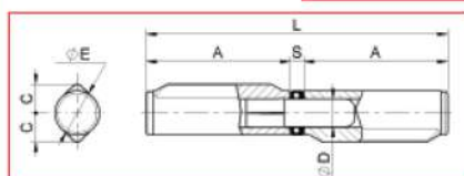
CERNIERA STAMPATA 2 ALI A COSTA, PERNO FISSO CUSCINETTO REGGISPINTA
