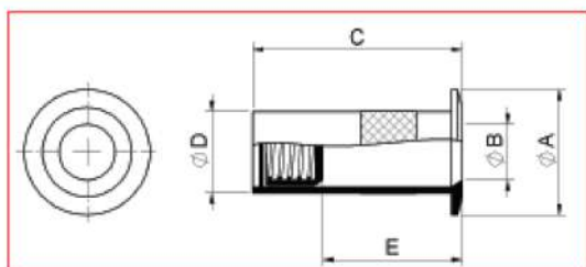
POZZETTO IN OTTONE CON MOLLA
