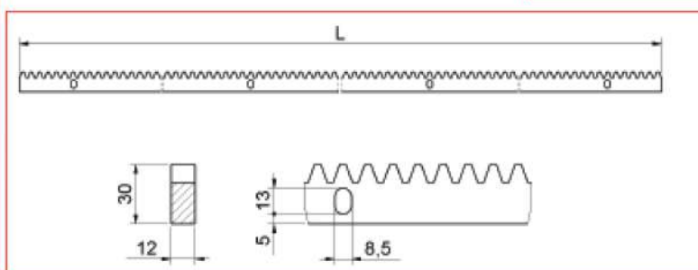
CREMAGLIERA RETTANGOLARE ZINCATA
