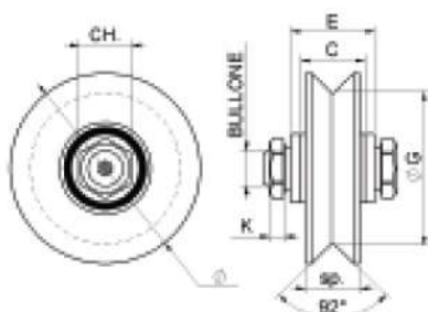
RUOTA GOLA A V A 2 CUSCINETTI, CON INGRASSATORE, ZINCATA
