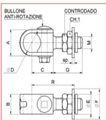
CARDINE A FASCETTA CON RONDELLA REGOLABILE E CONTRODADO PER TRONCHETTO ZINCATO
