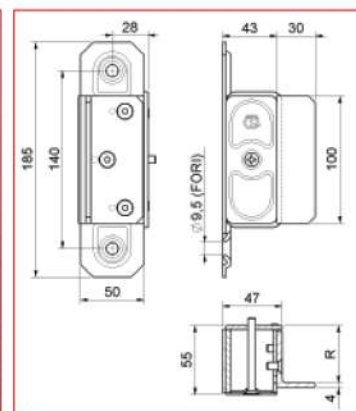
BATTENTE PORTA INCONTRO REGOLABILE PER ELETTRO-SERRATURE, ALI A FISSARE O SALDARE, ZINCATO
