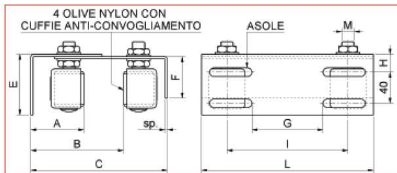
PIASTRA GUIDA REGOLABILE 4 OLIVE NYLON, ZINCATA
