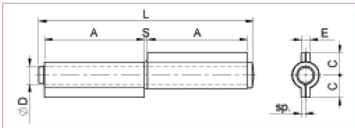
CERNIERA TRANCIATA 2 ALI, PERNO E RONDELLA SFILABILE IN ACCIAIO
