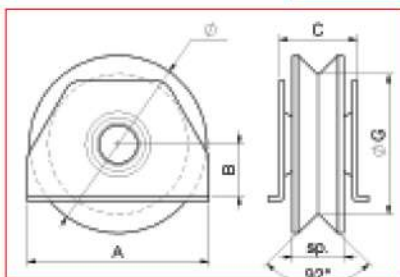
RUOTA GOLA A V A 2 CUSCINETTO, SUPPORTO LATERALE, ZINCATA
