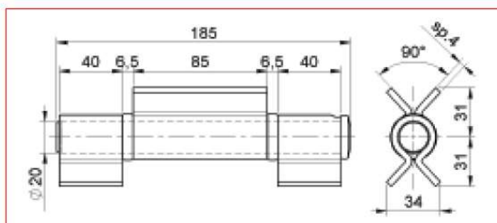
CERNIERA PER CANCELLI 3 ALI APERTE CON CUSCINETTI
