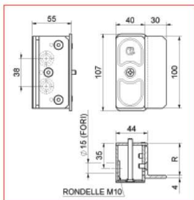
BATTENTE PORTA INCONTRO REGOLABILE PER ELETTRO-SERRATURE, ZINCATO
