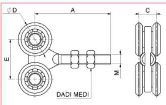
CARRELLO SCORREVOLE 4 CUSCINETTI, ZINCATO
