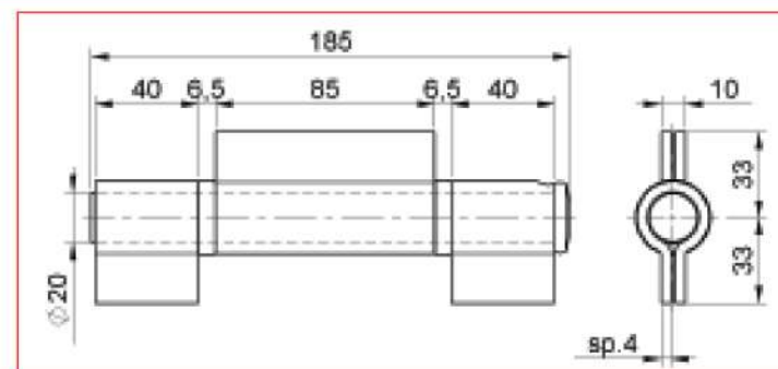
CERNIERA PER CANCELLI 3 ALI CHIUSE CON CUSCINETTI
