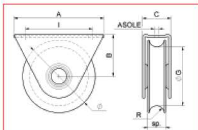
RUOTA GOLA TONDA CON SUPPORTO A CAVALLOTTTO A 1 CUSCINETTO, ZINCATA ART. M020 006 102 2 CUSCINETTI
