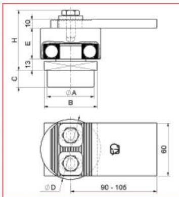
CARDINE REGOLABILE PER TUBOLARI CON CUSCINETTO, ZINCATO
