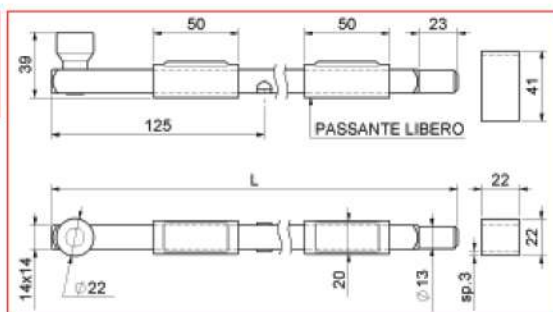
CATENACCIO VERTICALE 14x14 CON PUNTA TONDA, ZINCATO
